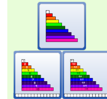
Jeu d'association (Nombres naturels)
